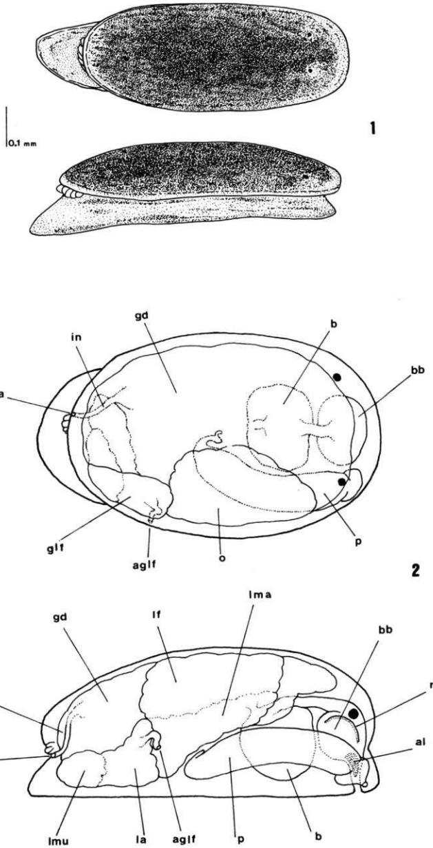
FIG. 1-2. — Runcina lenticula n. sp. : 1, vista dorsal y lateral de un animal vivo; 2, vista superior y lateral de la estructura interna.
