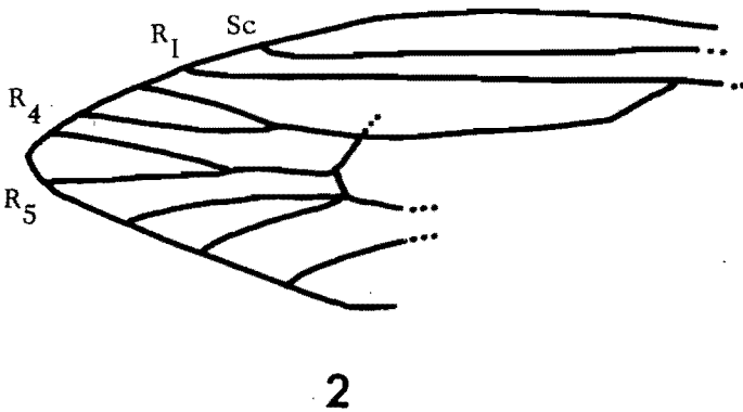
FIG. 2. Parasabatınca aftimacrai spec. nov., forewing venation.
