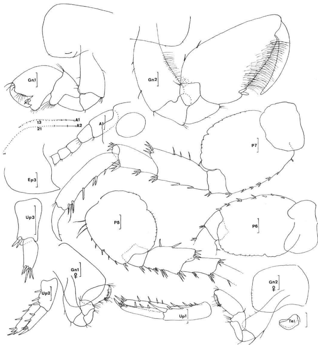
FIG. 17. — Hyale diploactyla Stebbing. Mâle et femelle, St. 15764, MONOD coll. Échelle 0,1 mm.
